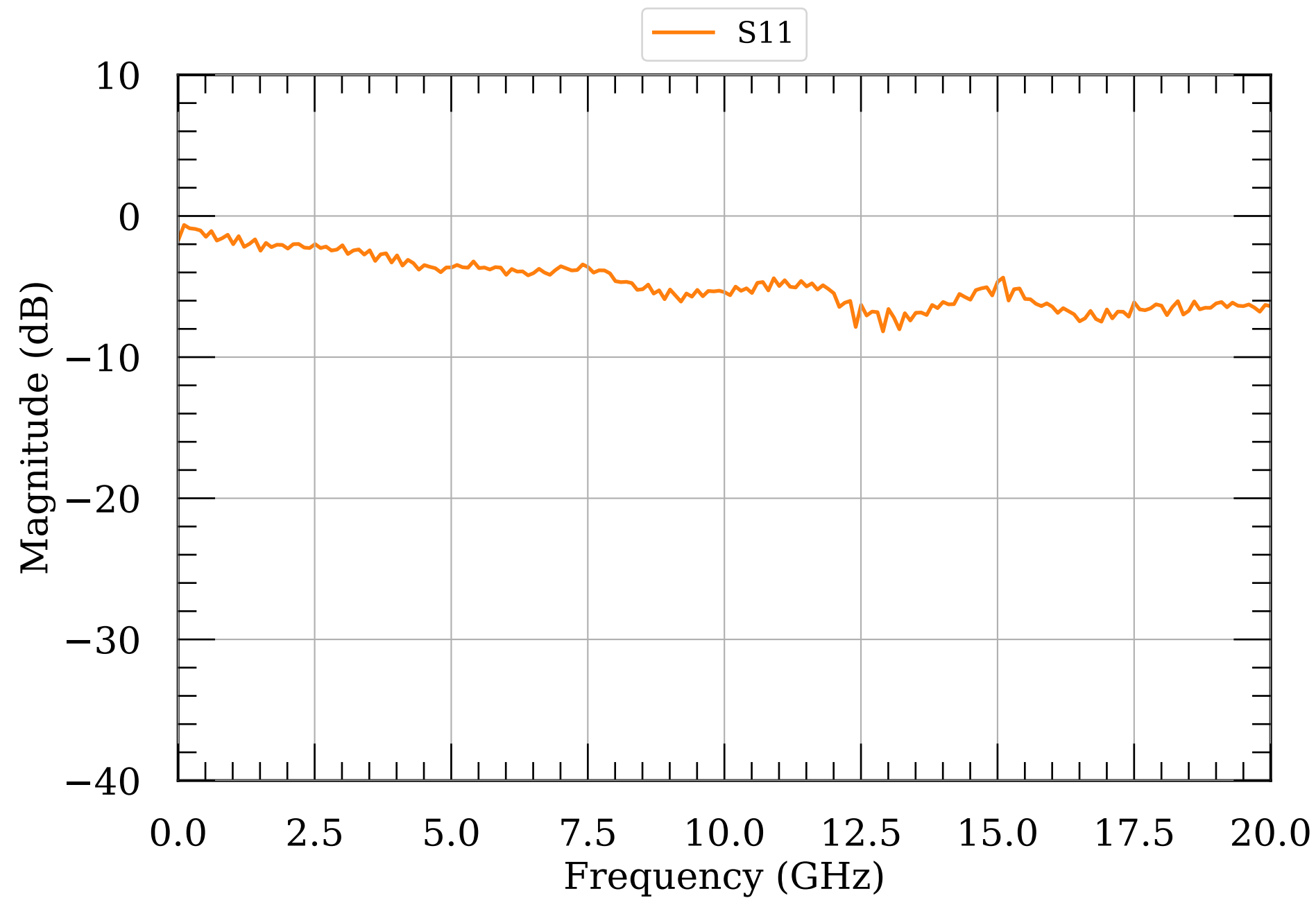
LNA S-params module021
